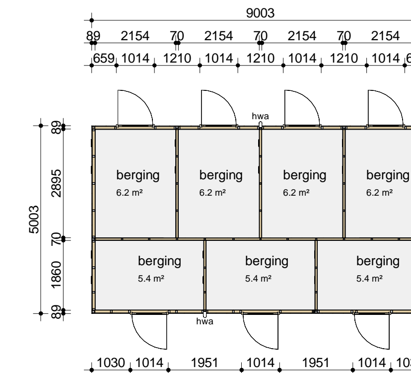
08_01 zevenvoudige berging
