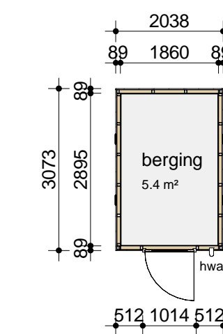
01_01 enkelvoudige berging
