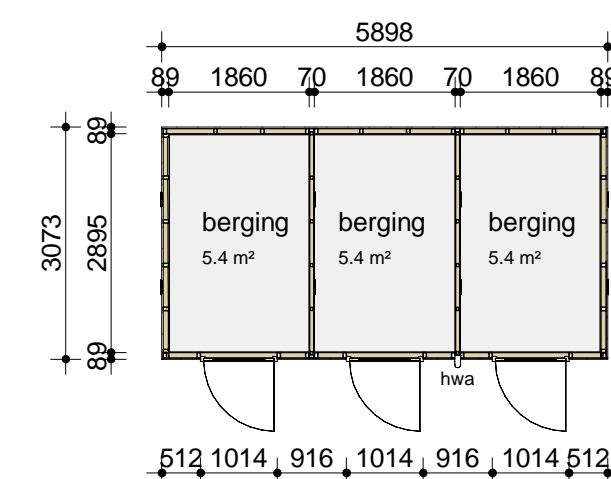
02_01 drievoudige berging
