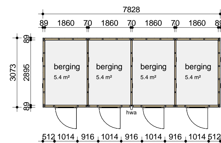
03_01 viervoudige berging
