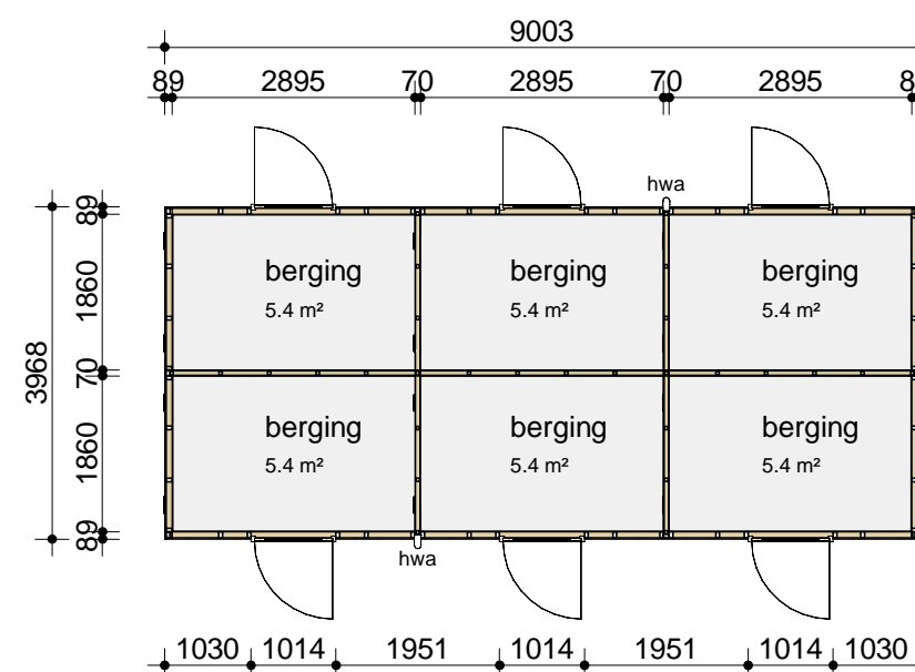
06_01 zesvoudige berging
