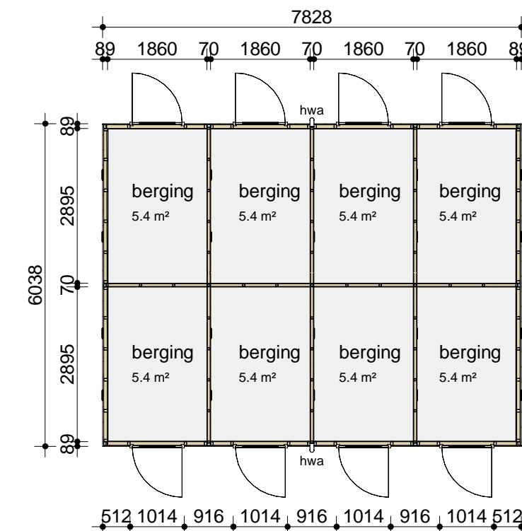
09_01 achttvoudige berging
