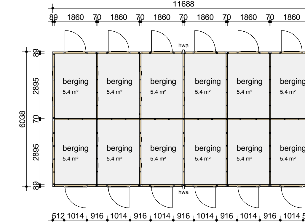
11_01 elfvoudige berging
