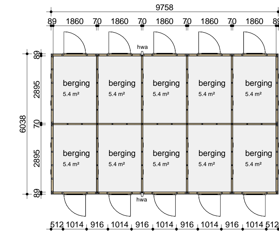
10_01 tienvoudige berging
