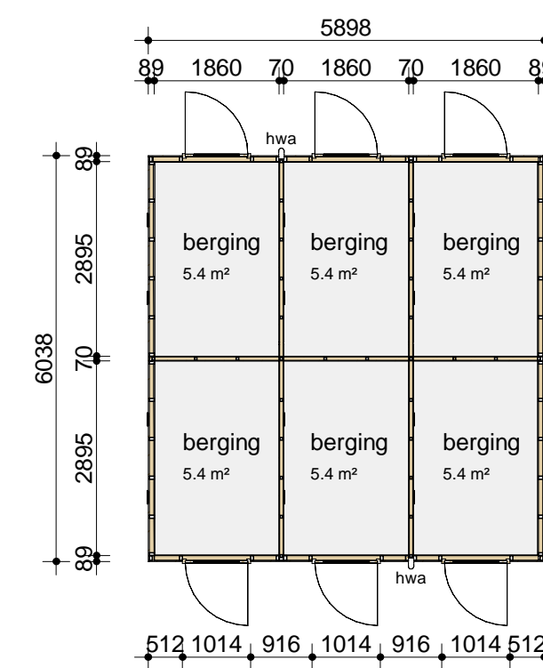
07_01 zesvoudige berging 2
