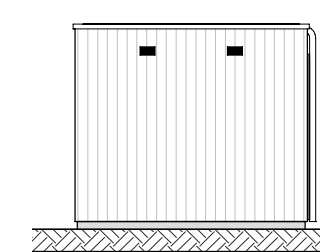
linkzijgevels
