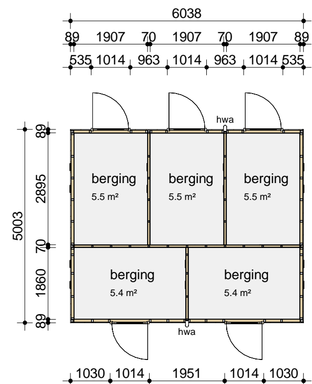
05_01 vijfvoudige berging
