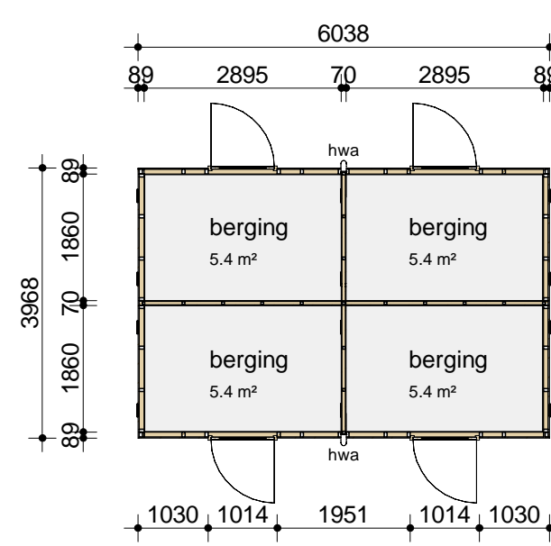
04_01 viervoudige berging 2
